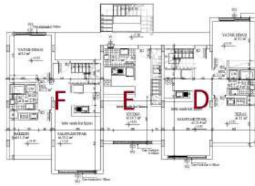
1. KAT PLANI
