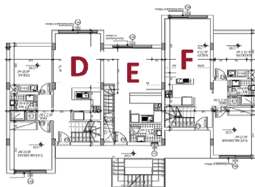
1. KAT PLANI
